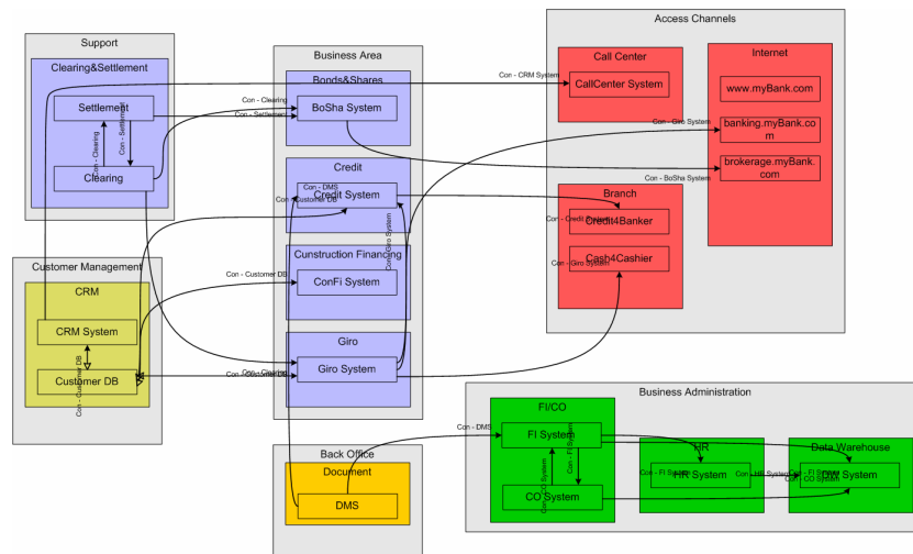
Abbildung 4: Softwarekarte vom Typ Clusterkarte
