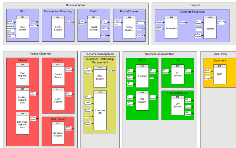
Abbildung 1: Softwarekarte mit logischen Einheiten und Verbindungen
