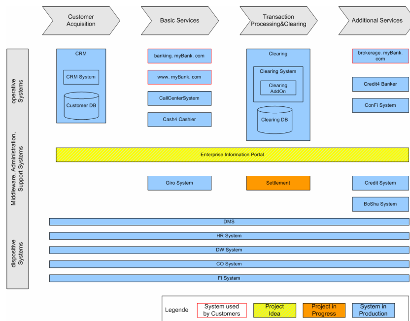
Abbildung 7: Prozessunterstützungskarte mit Systemtypen
