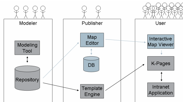
Abbildung 10: Architektur eines Werkzeuges zur Softwarekartographie
