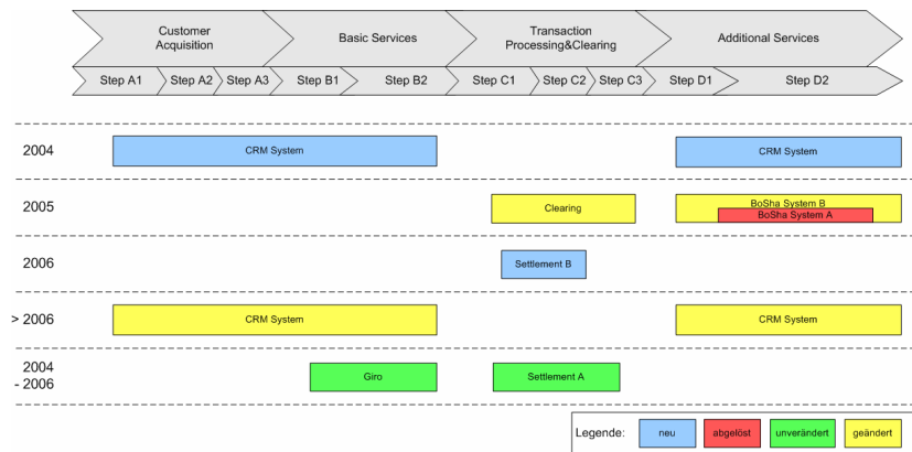
Abbildung 6: Prozessunterstützungskarte mit Evolutionsschritten
