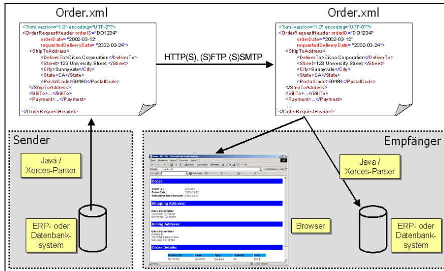
Abbildung 1: Einfache Anwendung von XML/EDI
