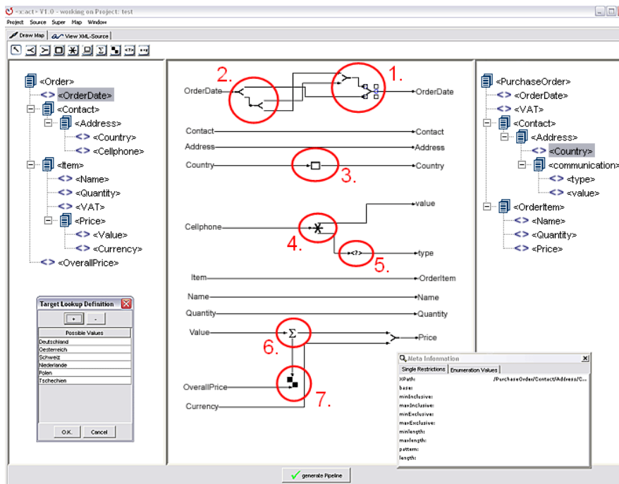
Abbildung 6: Screenshot des <x:act> Mappers
