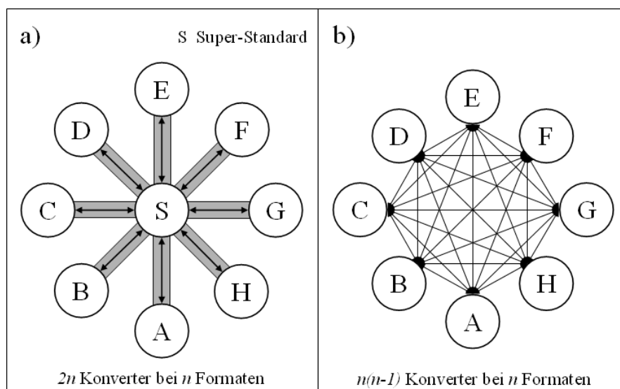
Abbildung 3: Konvertierung mittels eines intermediären Formats (a) und mittels eines vollständig vermaschten Netzes (b) 3
