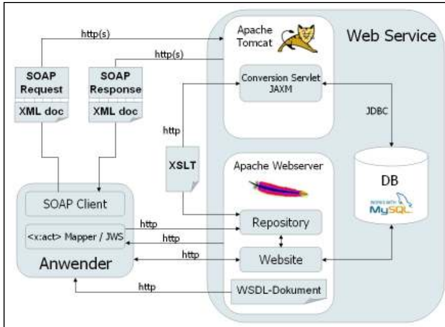
Abbildung 7: Die Architektur des &lt;x:act&gt; Webservice
