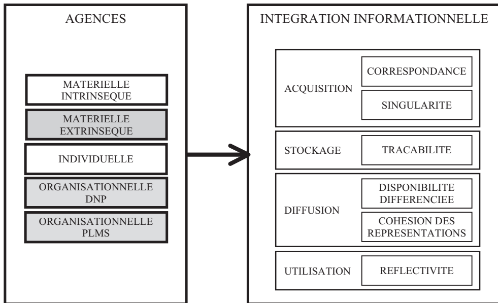
Figure 1. Modèle conceptuel.
