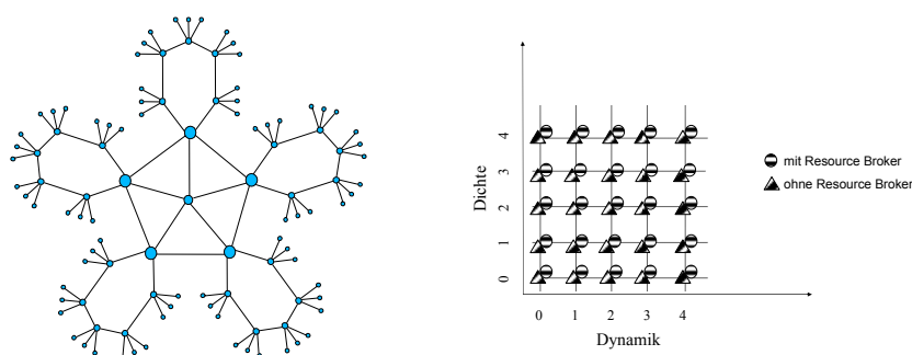
Abbildung 3a/b: Netztopologie und Experimentraum mit den Dimensionen Dichte und Dynamik
