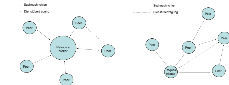
Abbildung 1a/b: Ablauf zentraler und dezentraler Dienstfindung und -selektion
