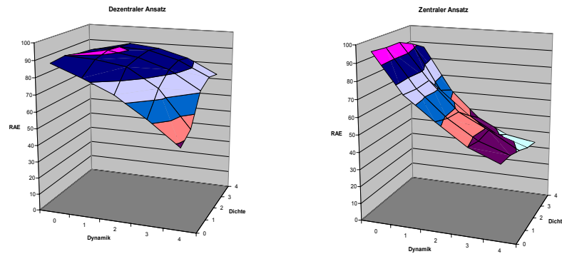
Abbildung 4a und b: Gemessene Allokationseffizienz ohne und mit Resource Broker
