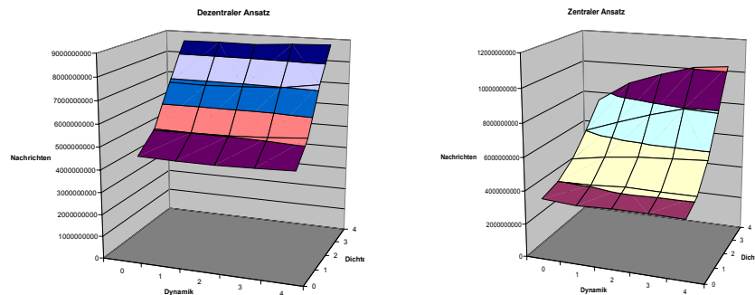
Abbildung 5a und b: Anzahl der Kontrollnachrichten ohne und mit Resource Broker
