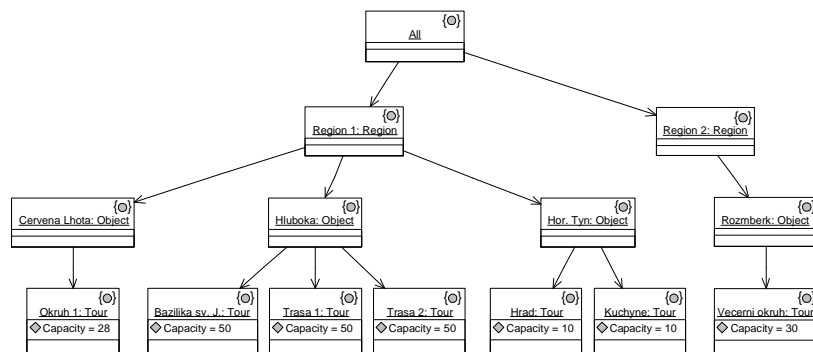
Abbildung 7: Beispiel eines Dimensionenbaums
