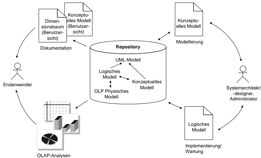
Abbildung 8: Metadatenfluß und -zugriff mit Hilfe von ADAPTEd-UML
