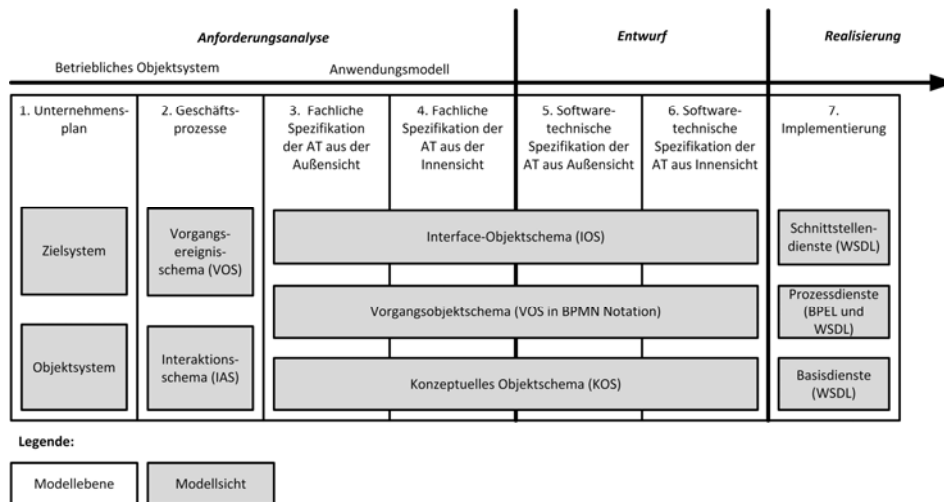
Abbildung 3: Modellarchitektur
